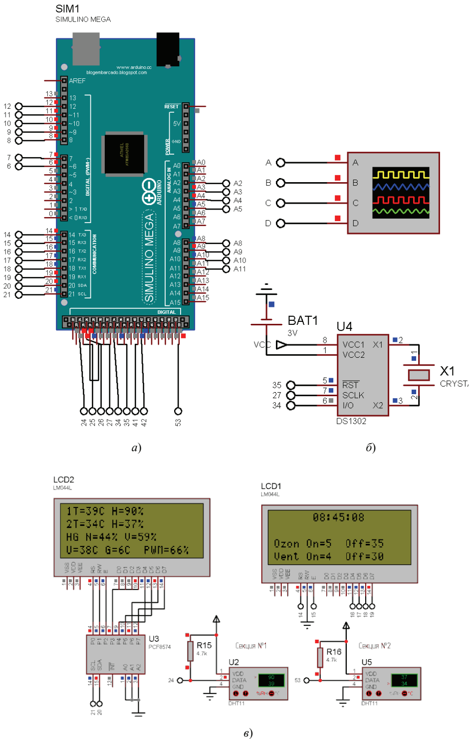
Рис. 2. Моделирование работы схемы при условиях: 2T < U ; 2H < HG , текущее время 8:45:08 (начало):
